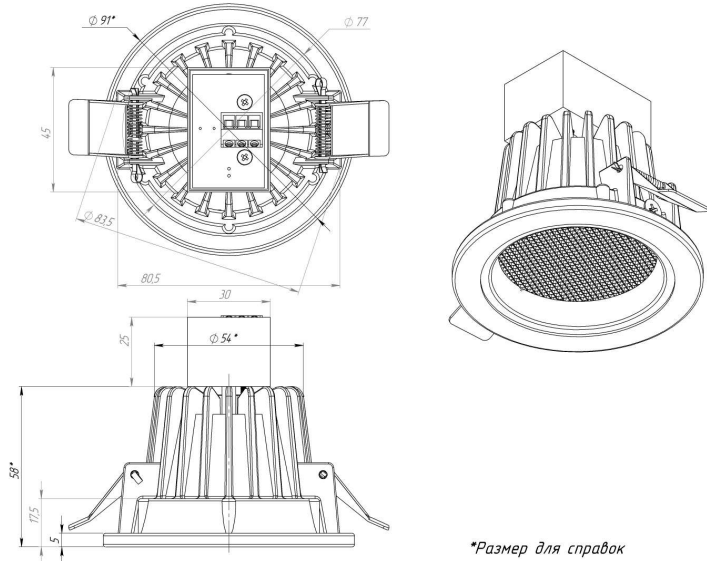
Рисунок 1 Светильник « Radian 12».
