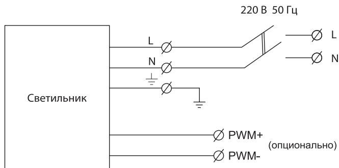
Рисунок 2 . Схема подключения светильника
